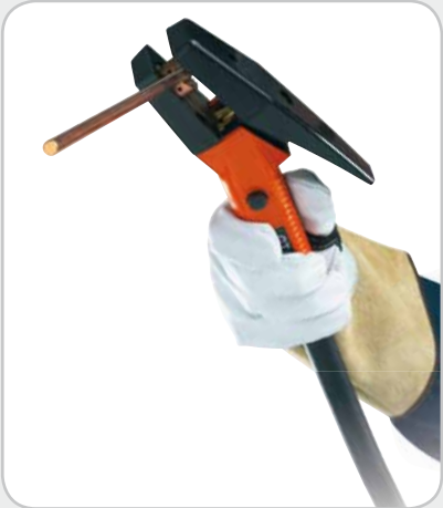
Il supporto per l'elettrodo della scriccatura GT4000 è progettato per essere utilizzato con KempGouge ed è adatto per gli elettrodi rotondi o per quelli piatti.
