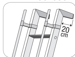
Distanziali saldati
